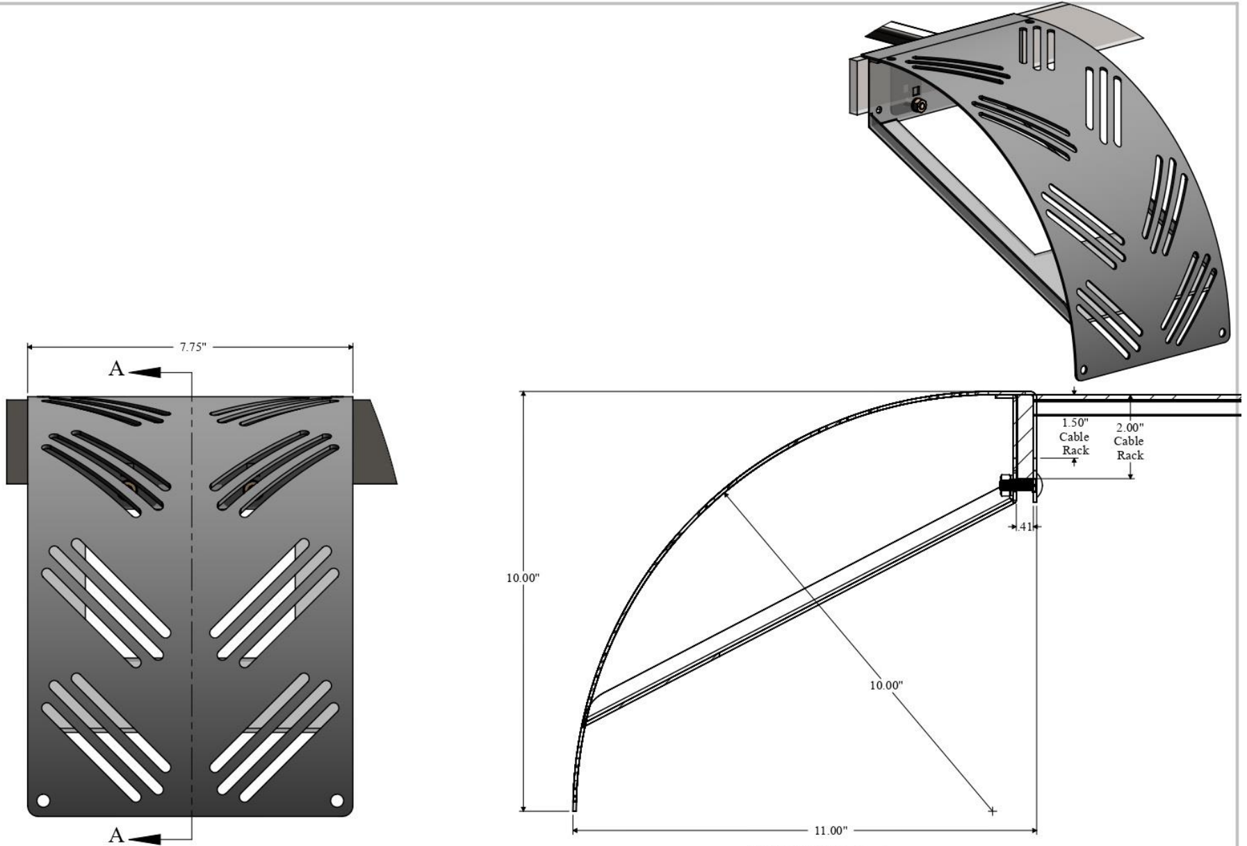
SECTION A-A
