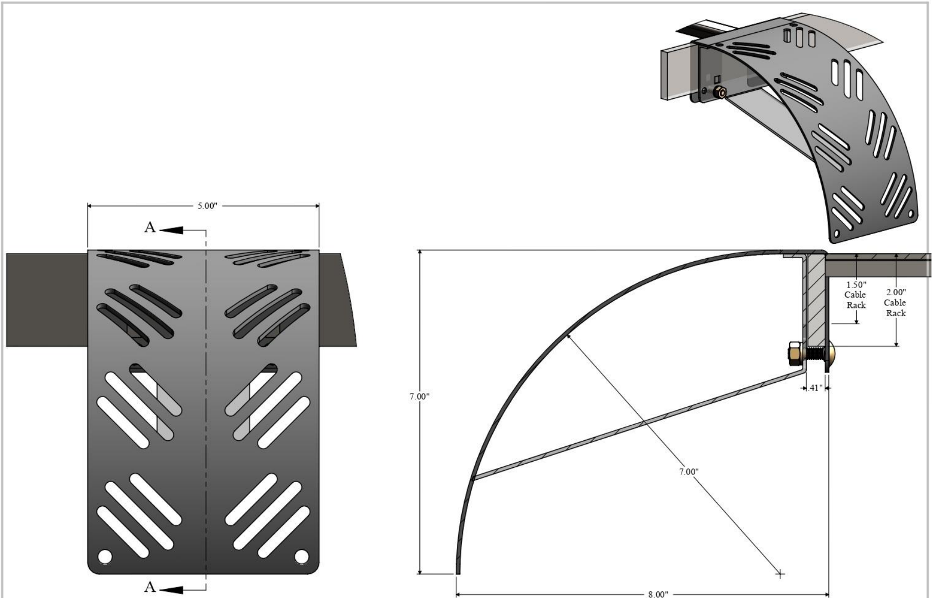
SECTION A-A
